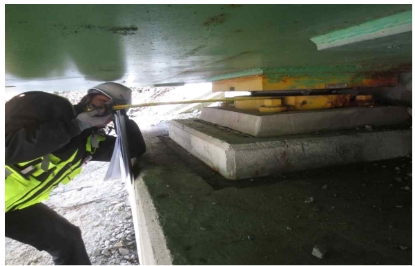
교량받침장치 연단거리 측정
